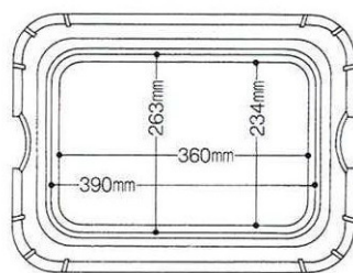
カバー (No.10-173-134)
